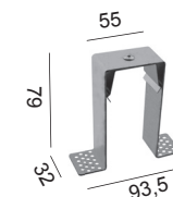
Staffa di fissaggio per cartongesso Plasterboard bracket
