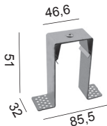
Staffa di fissaggio per cartongesso Plasterboard bracket
